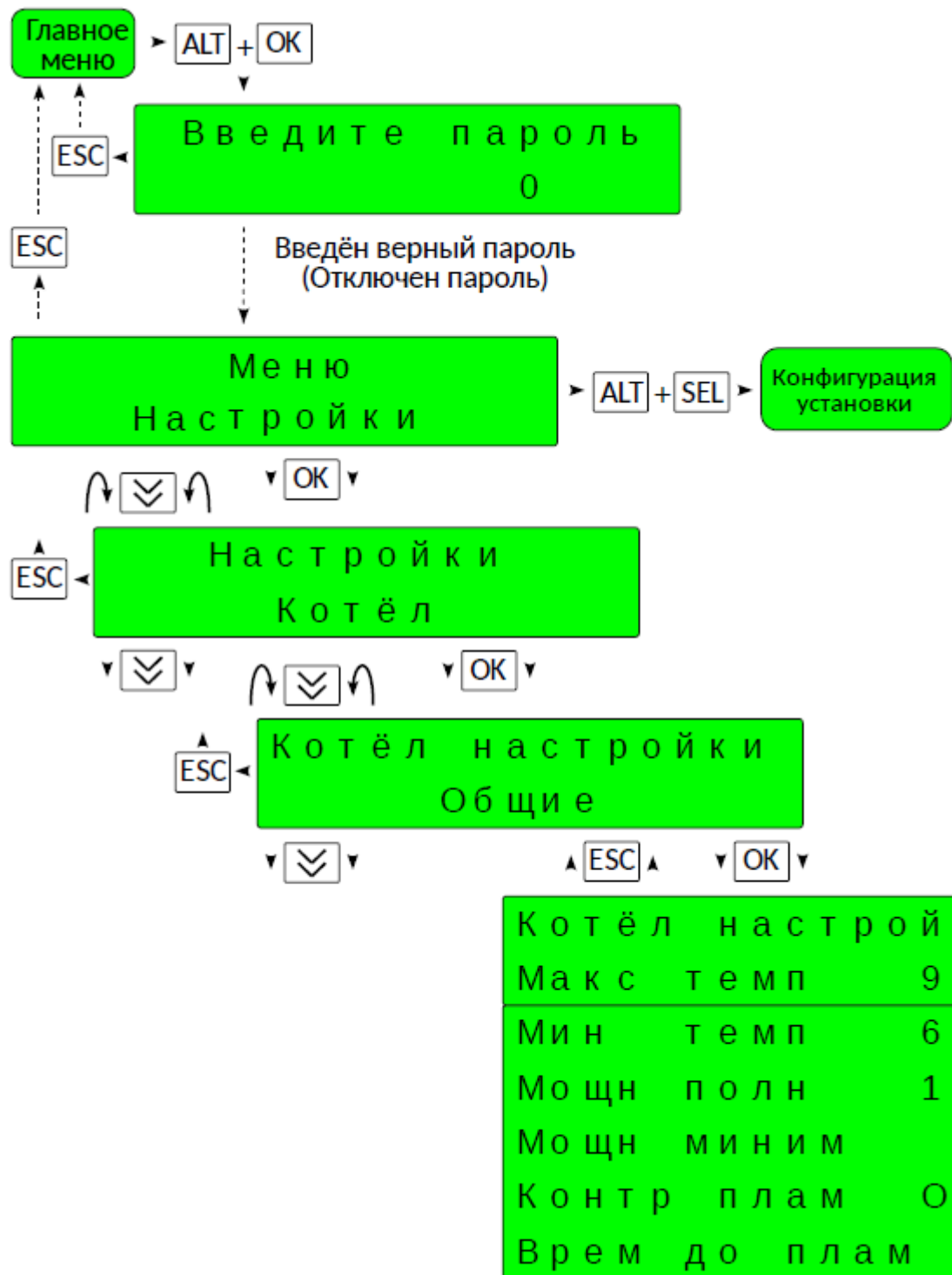
Рисунок 4 – Меню «Настройки котел»
